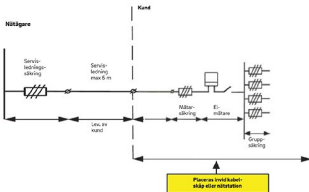
Figur 3: Byggkraft <63 A, exempel
