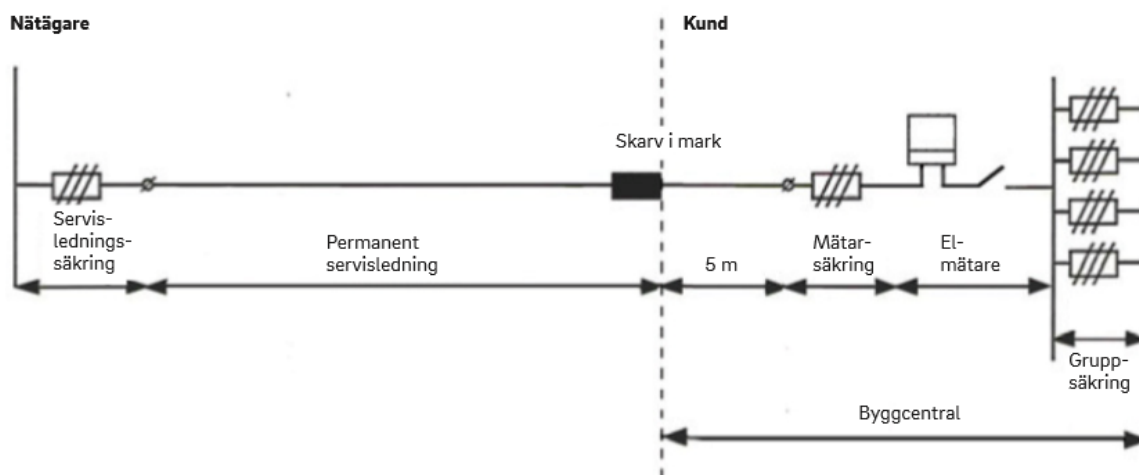
Figur 5: Byggekraft <63, exempel 4, byggekraft på redan befintlig anläggning, servis i tomtgräns.
