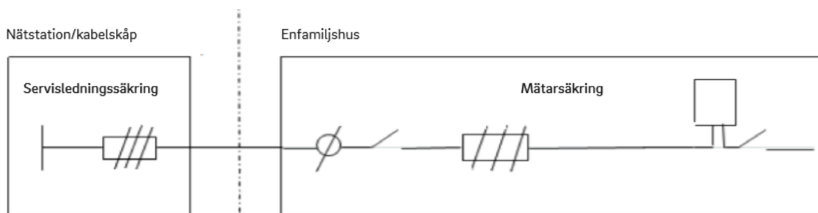
Figur 8: Skiss på anläggning med en mätarplats.
