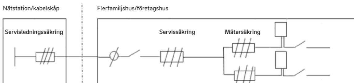
Figur 7: Skiss på anläggning med flera mätarplatser.
