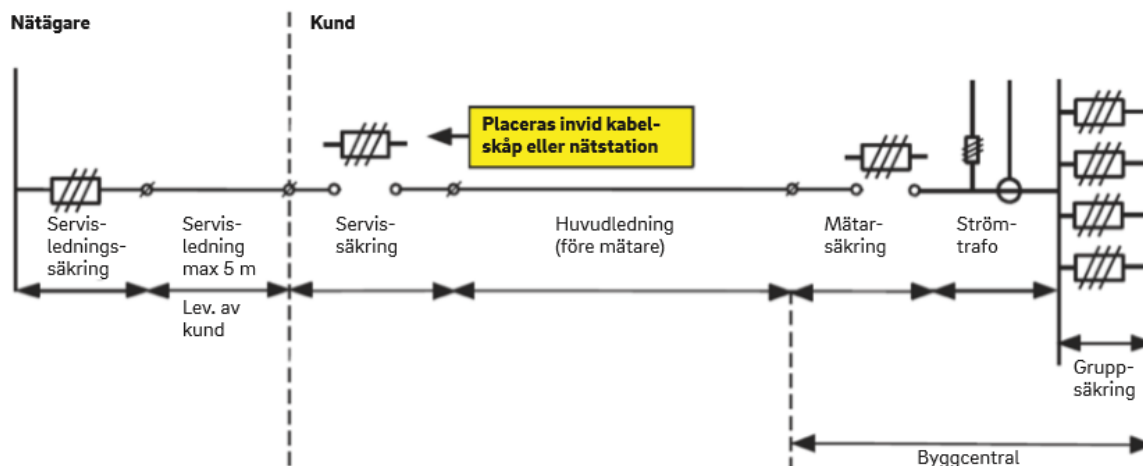
Figur 4: Byggekraft >63 A, exempel
